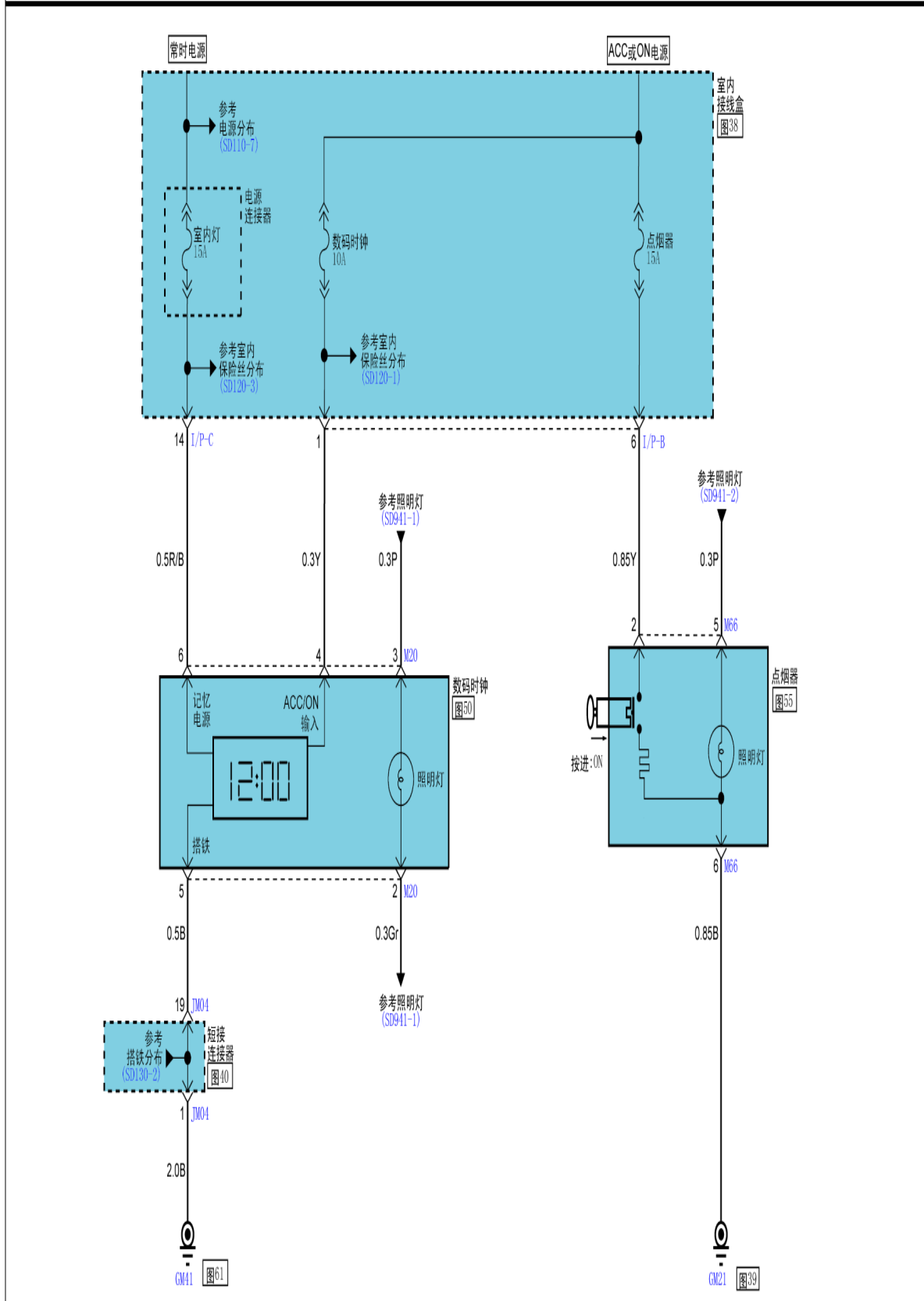
时钟&amp;点烟器(电源插座) (1)
